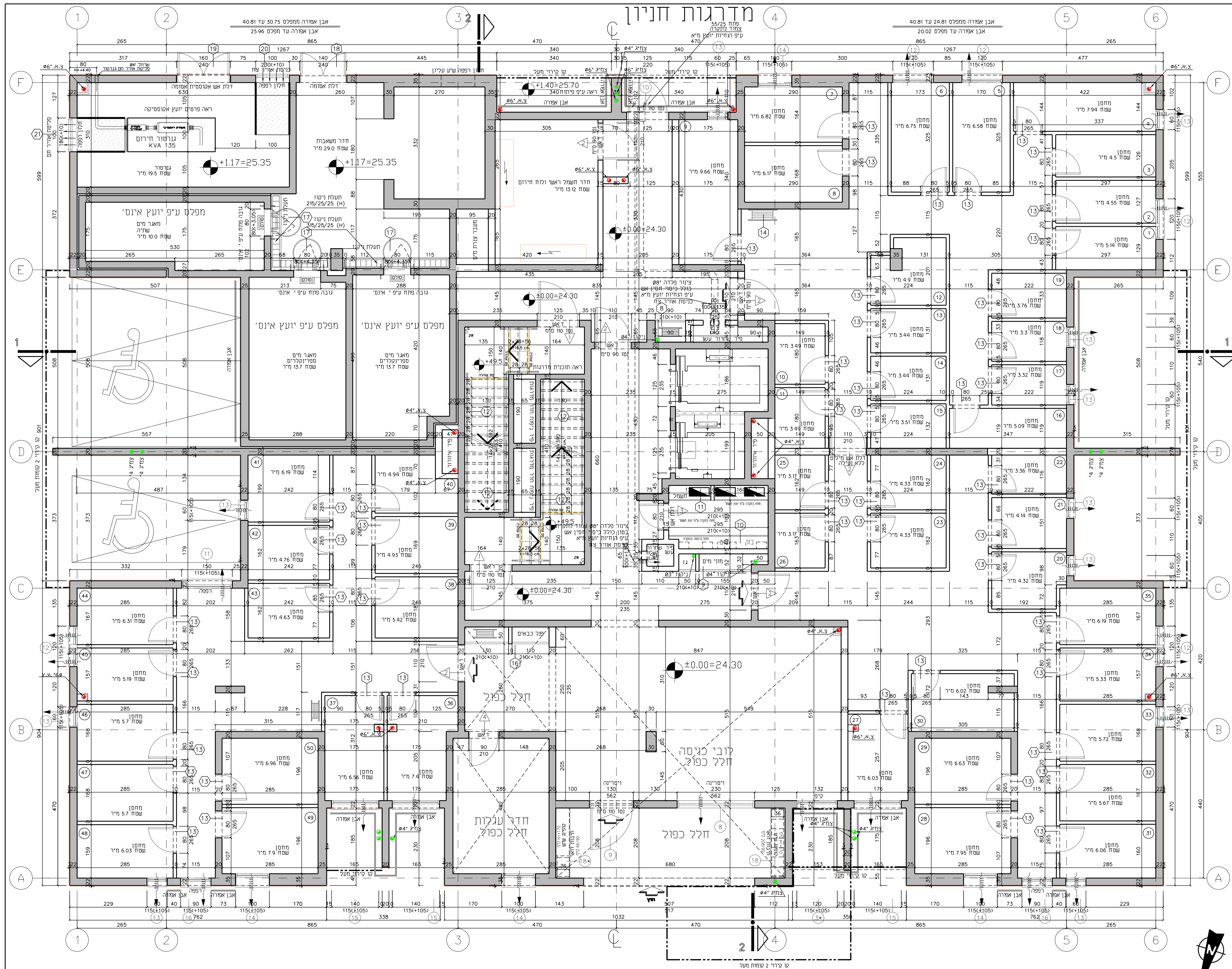
קומת קרקע מפלס 0.00
