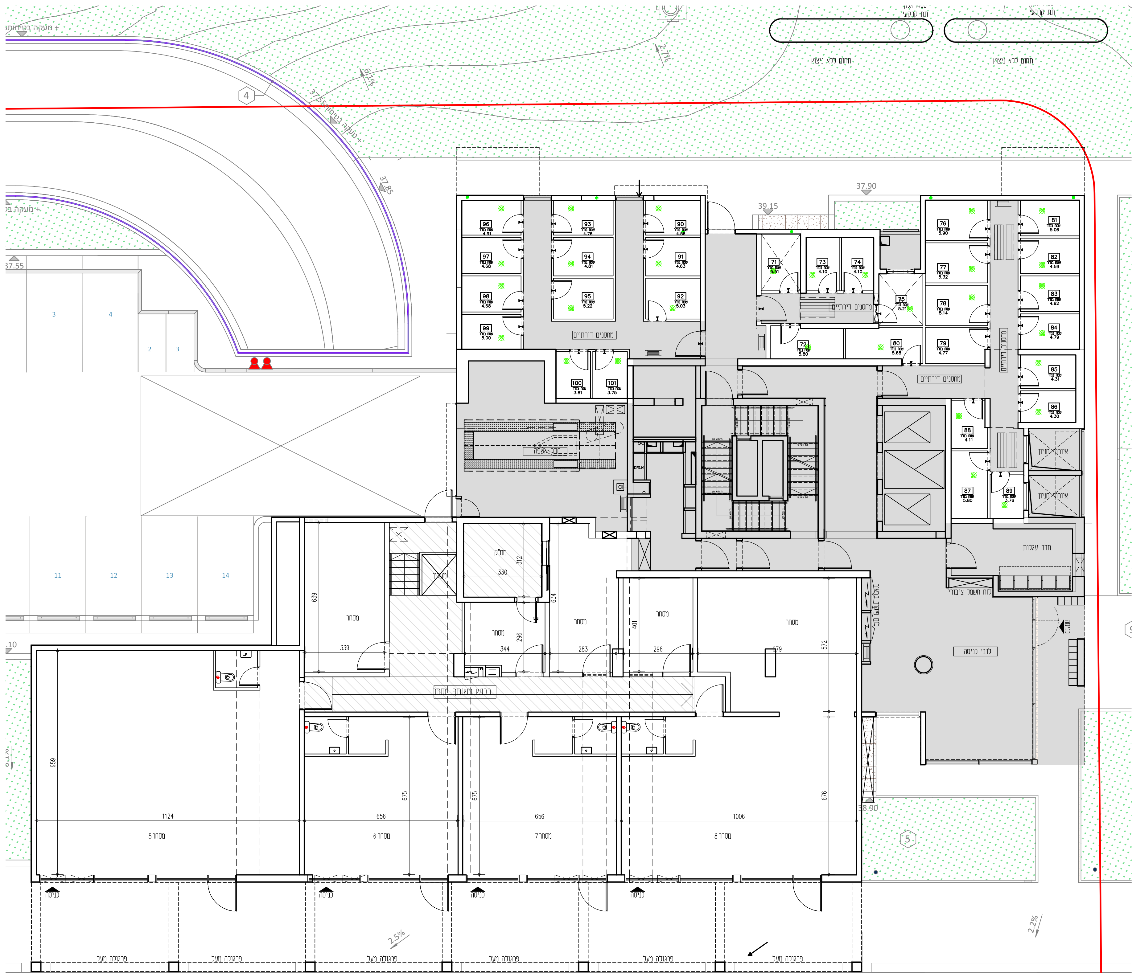
קומת קרקע - 1
